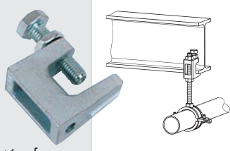
Tartópófa 0862 200 002
