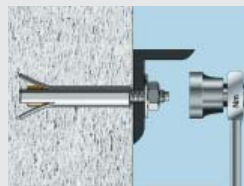
Fix-anker W-FAZ/S 0904 52. ...
