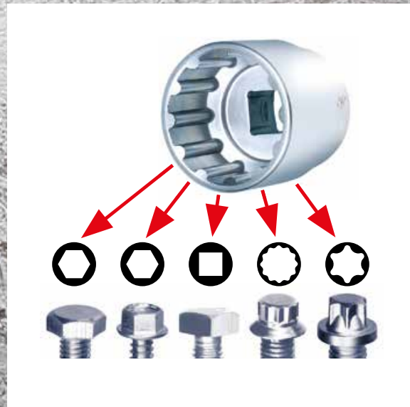
MULTIPROFIL
